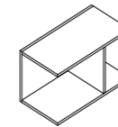
Nicho fixo H *com fechamento posterior *capacidade de carga 20kg FLO7013 - 700 X 368 X 388
