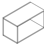
Nicho fixo *com fechamento posterior *capacidade de carga 15kg FLO7006 - 700 X 368 X 388
