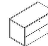
Nicho com gaveta *com 02 gavetas *capacidade de carga 30kg FLO7017 - 700 X 388 X 388
